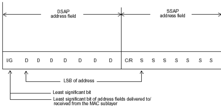
Fig. 3-2 SAP Format
